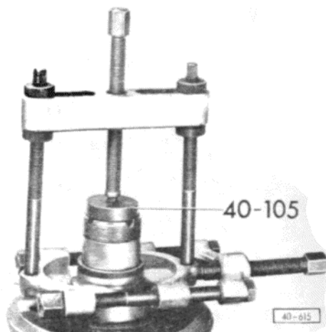
Abb. 4 Lagerinnenring abziehen
