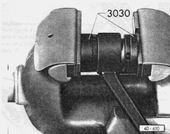
Abb. 3 Gummimetallager für Querlenker zwischen Schraubstockbacken einpressen
