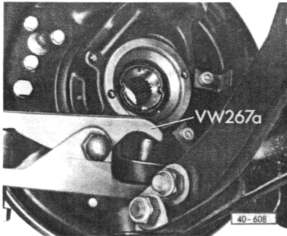
Abb. 1 Radlagergehäuse vom Führungsgelenk abdrücken
