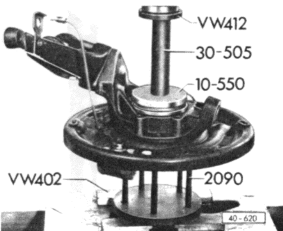
Abb. 9 Inneren Dichtring innen einpressen Vorher Sicherungsring innen einbauen.
