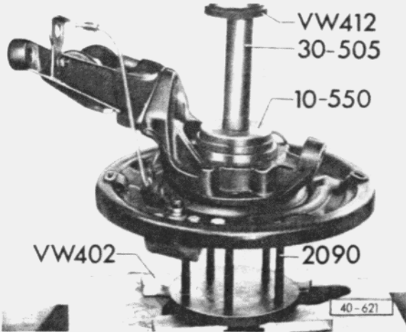
Abb. 8 Radlager aus- und einpressen Vor dem einpressen Sicherungsring außen einbauen.
