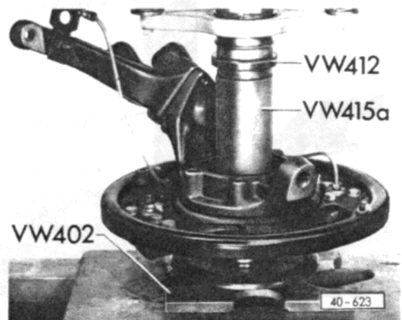
Abb. 12 Radnabe einpressen
