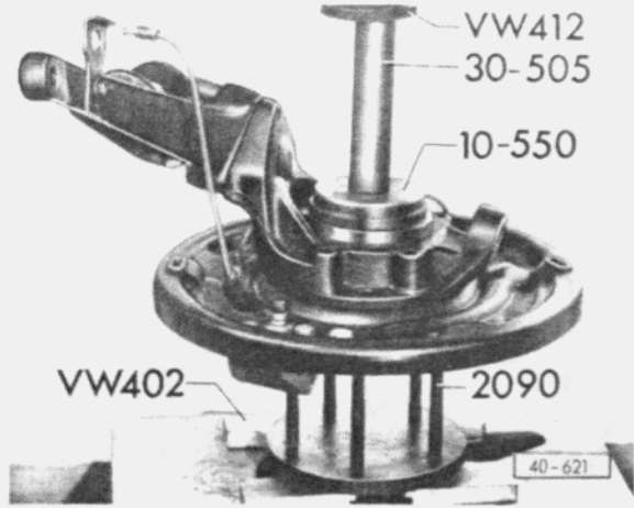
Abb. 10 Äußeren Dichtring innen einpressen
