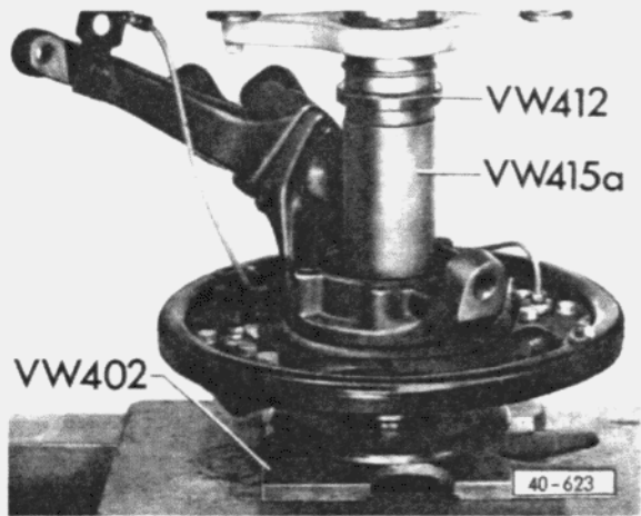
Abb. 12 Radnabe einpressen
