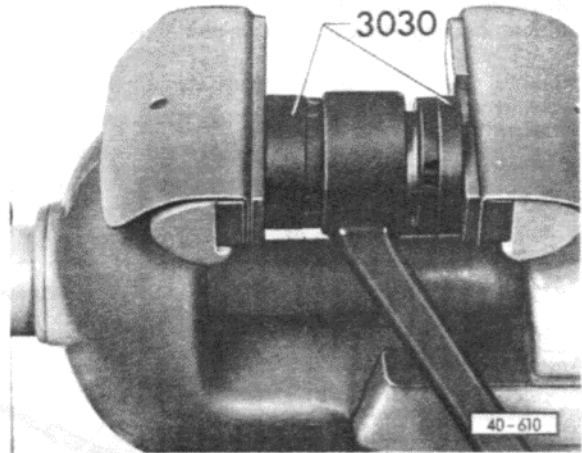
Abb. 4 Gummimetallager für Querlenker zwischen Schraubstockbacken einpressen
