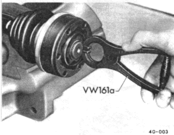
Abb. 2 Sicherungsring aus- bzw. einbauen
