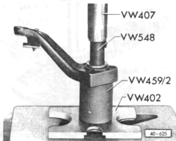
Abb. 14 Buchsen aus Lenkspurhebel auspressen
