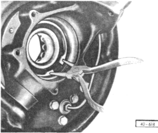
Abb. 7 Sicherungsring ausbauen
