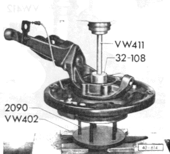
Abb. 3 Radnabe auspressen
