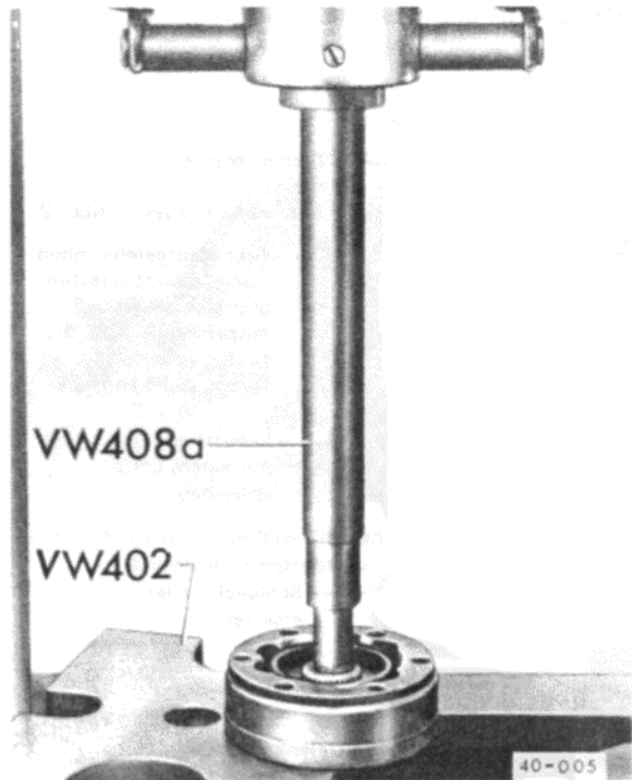
Abb. 3 Inneres Gelenk abpressen Dabei Kugelnabe abstützen.
