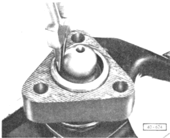
Abb. 13 Sicherungsring für Lenkspurhebel aus- und einbauen
