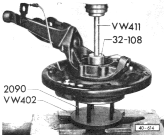
Abb. 3 Radnabe auspressen
