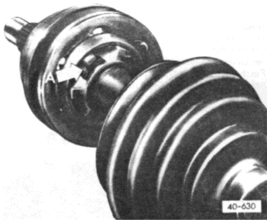
Abb. 1 Äußeres Gelenk ausbauen Sicherungsring (Pfeil A) spreizen, und gleichzeitig das Gelenk mit einem Plastikhammer von der Welle abtreiben.
