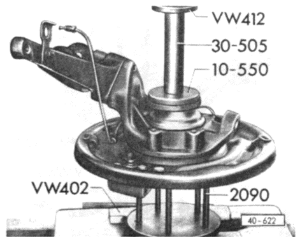
Abb. 11 Äußeren Dichtring innen mit der Mutter für die Radnabe bis zum Anschlag nachpressen
