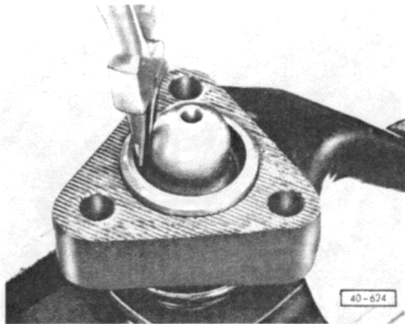
Abb. 13 Sicherungsring für Lenkspurhebel aus- und einbauen
