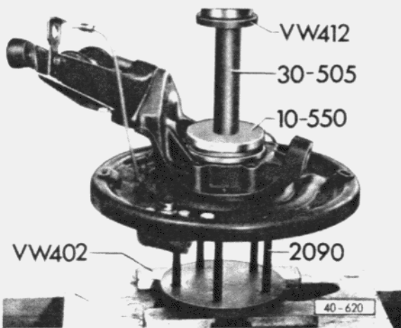
Abb. 9 Inneren Dichtring innen einpressen Vor dem einpressen Sicherungsring innen einbauen.
