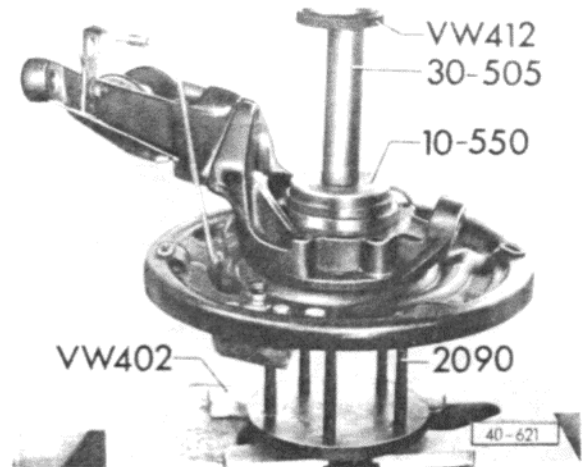
Abb. 10 Äußeren Dichtring innen einpressen
