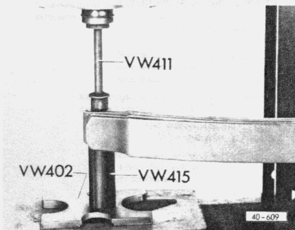
Abb. 2 Gummimetallager für Blattfeder aus- und einpressen
