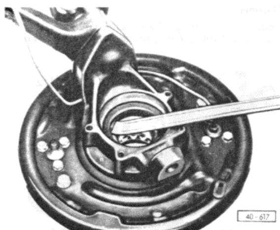
Abb. 6 Inneren Dichtring innen ausheben
