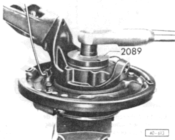
Abb. 2 Mutter für Radnabe lösen bzw. festziehen
