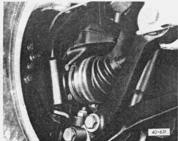
Abb. 4 Befestigung Lenkanschlag
