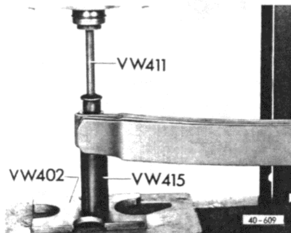
Abb. 3 Gummimetallager für Blattfeder aus- und einpressen
