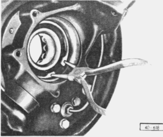
Abb. 7 Sicherungsring ausbauen
