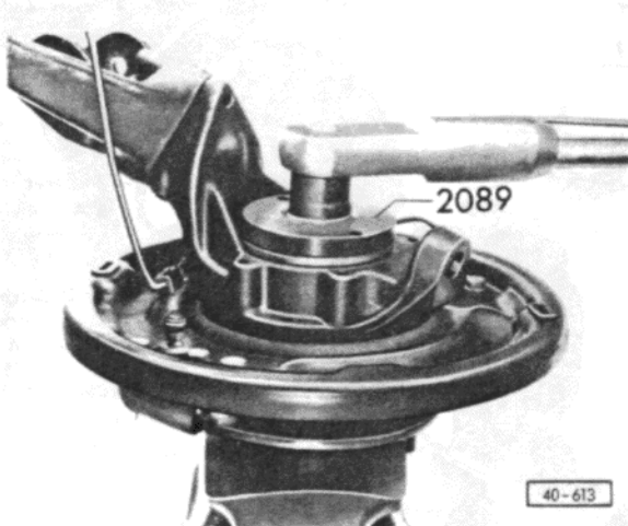
Abb. 2 Mutter für Radnabe lösen bzw. festziehen
