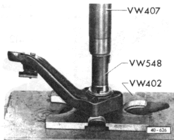
Abb. 15 Obere Buchse für Lenkspurhebel bündig einpressen
