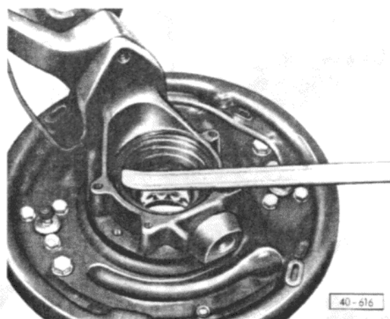
Abb. 5 Äußeren Dichtring innen ausheben
