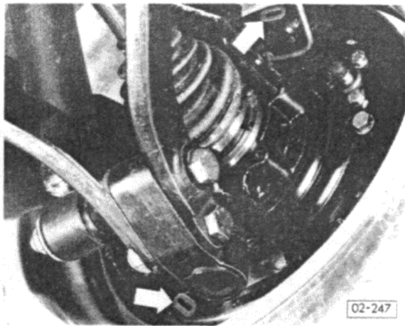
Abb. 1 Bremsbelagdicke prüfen Verschleißgrenze: 2,5 mm
