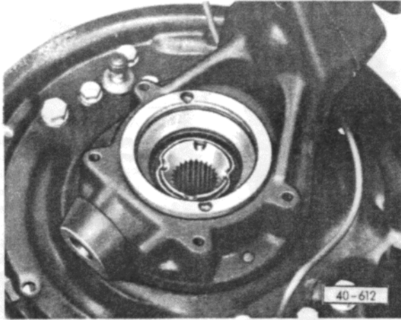
Abb. 1 Mutter für Radnabe
