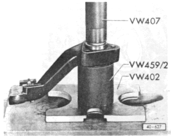
Abb. 16 Untere Buchse für Lenkspurhebel bis zum Anschlag einpressen
