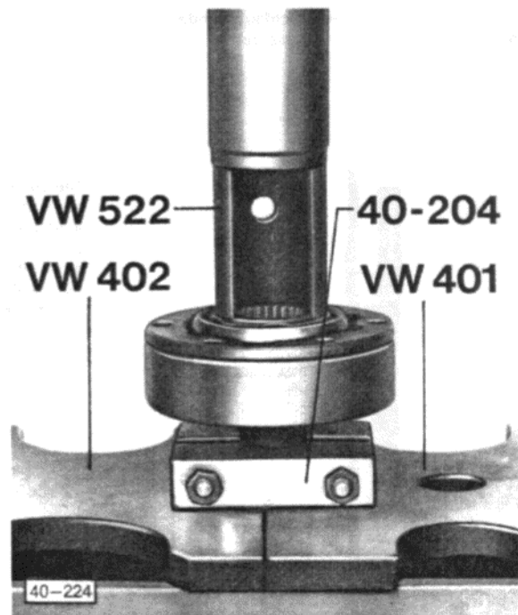
Abb. 4 Inneres Gelenk aufpressen Gelenk bis Anschlag aufpressen. Sicherungsring einbauen.
