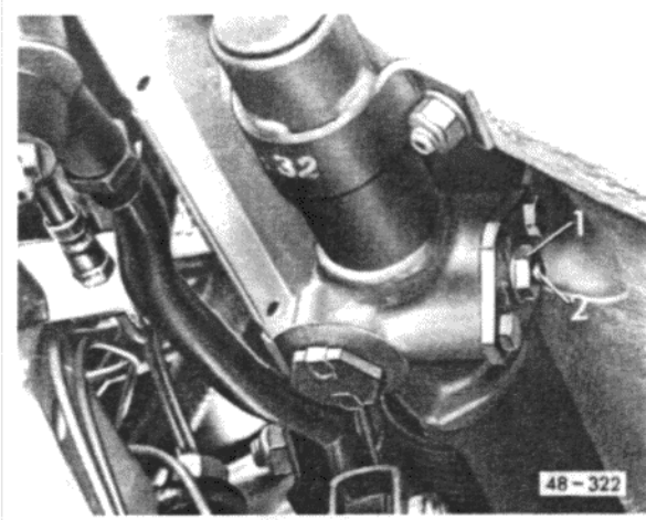
Abb. 1 Lenkungsspiel einstellen
