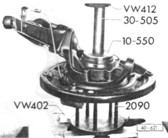
Abb. 8 Radlager aus- und einpressen Vorher Sicherungsring außen einbauen.
