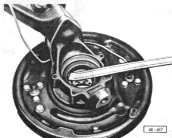
Abb. 6 Inneren Dichtring innen ausheben
