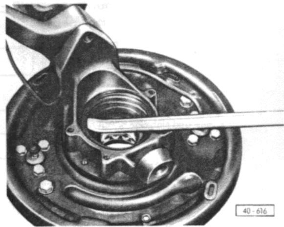
Abb. 5 Äußeren Dichtring innen ausheben
