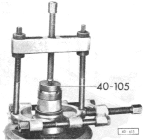
Abb. 4 Lagerinnenring abziehen
